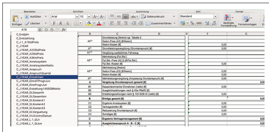
Abb. 2: Referenzierung von Datenbankfeldern unter Verwendung von Excel-Feldnamen.
